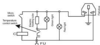
1 фаза 220В
